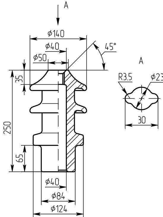
ИПТ-10/630 А 01 чертеж ИВЕЮ.757523.149 креслення
